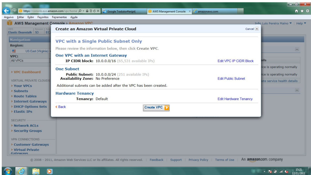
Ilustração 47: Criação de VPC no Amazon Web Services.
