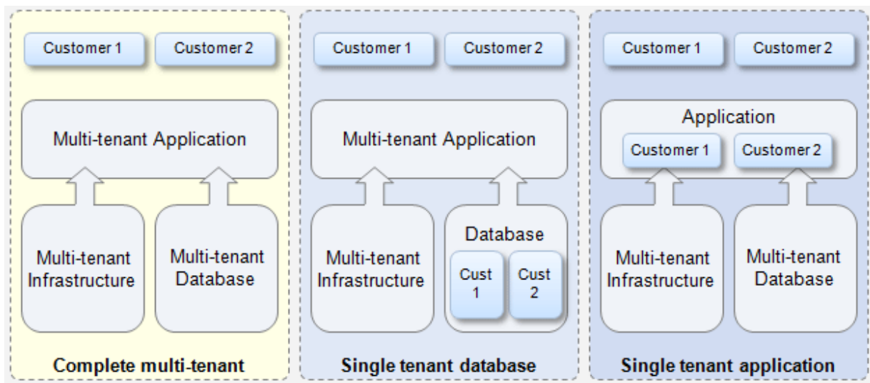
Ilustração 6 : Diagrama multitenancy (PERERA,2011)
