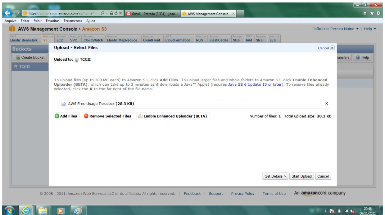
Ilustração 50: Salvando arquivos no Amazon S3.
