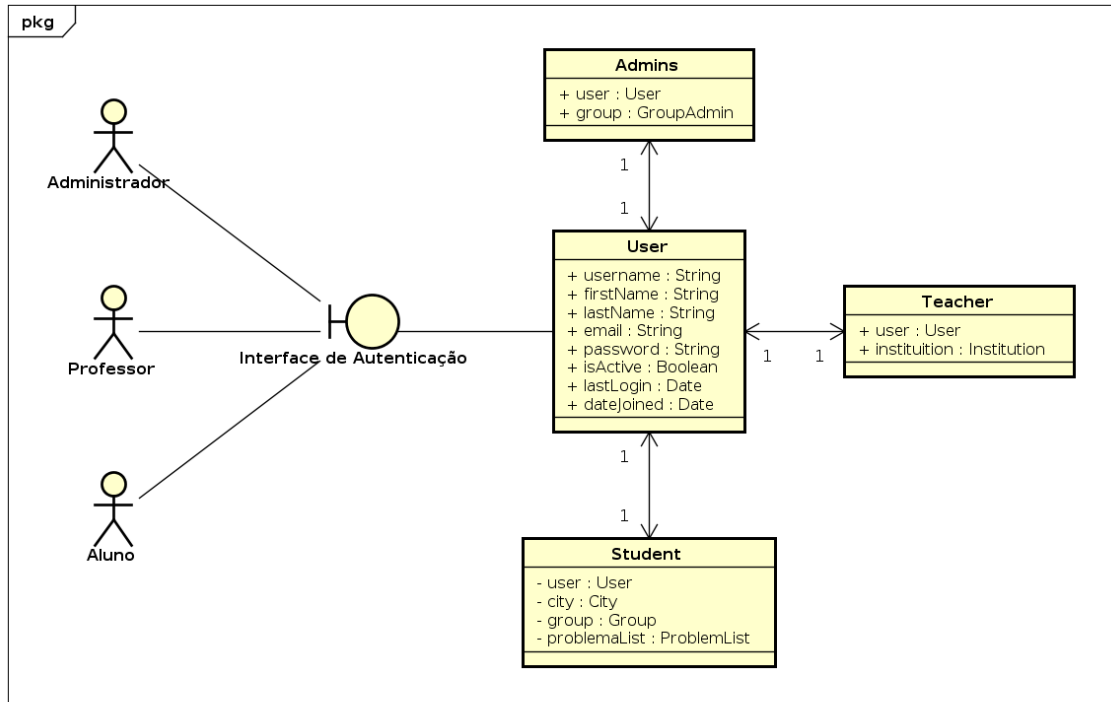
Figura 4.37: Diagrama de Robustez de Autenticação
