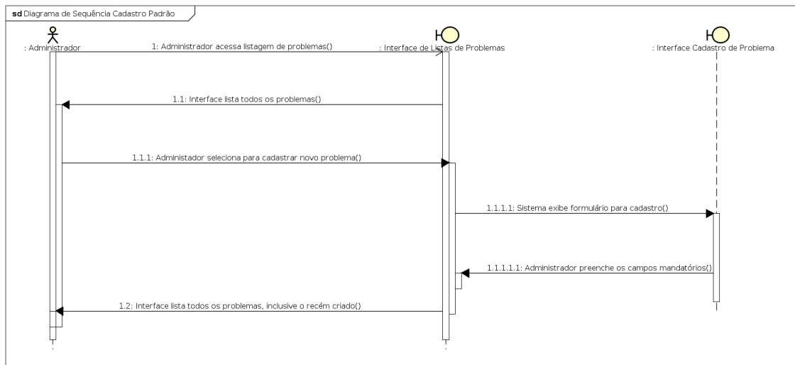
Figura 4.67: Diagrama de Sequência de Cadastro e Edição de Problemas
