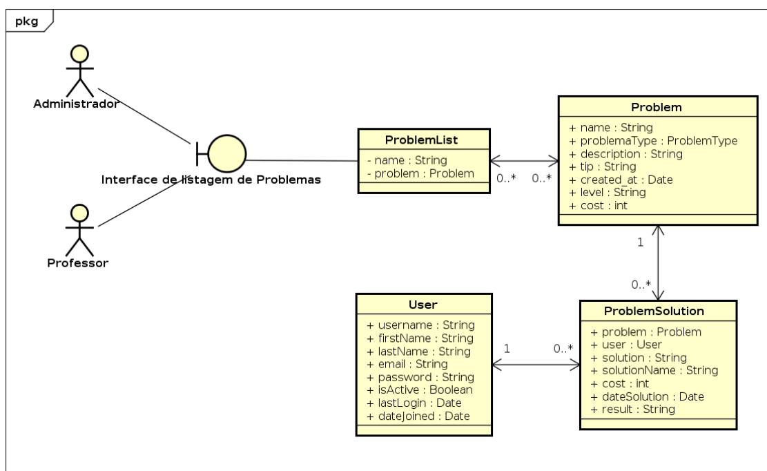
Figura 4.39: Diagrama de Robustez de Problemas
