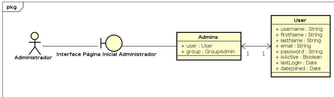
Figura 4.38: Diagrama de Robustez de Boas Vindas Administrador
