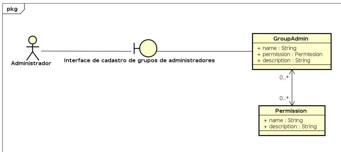
Figura 4.62: Diagrama de Robustez de Cadastro e Edição de Grupos de Administradores
