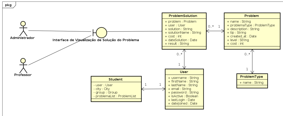
Figura 4.44: Diagrama de Robustez de Visualização de Solução partindo da listagem de Problemas
