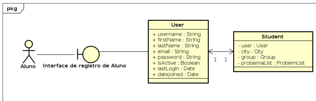
Figura 4.36: Diagrama de Robustez de Cadastro de Aluno
