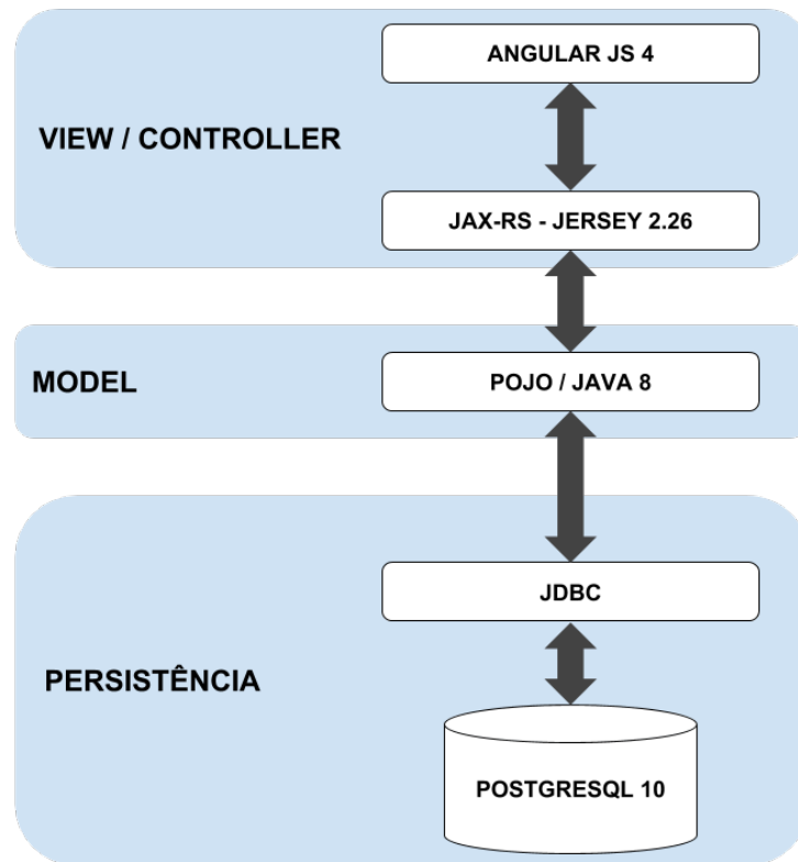
Figura 4.69: Arquitetura do Software do Portal de Algoritmos
