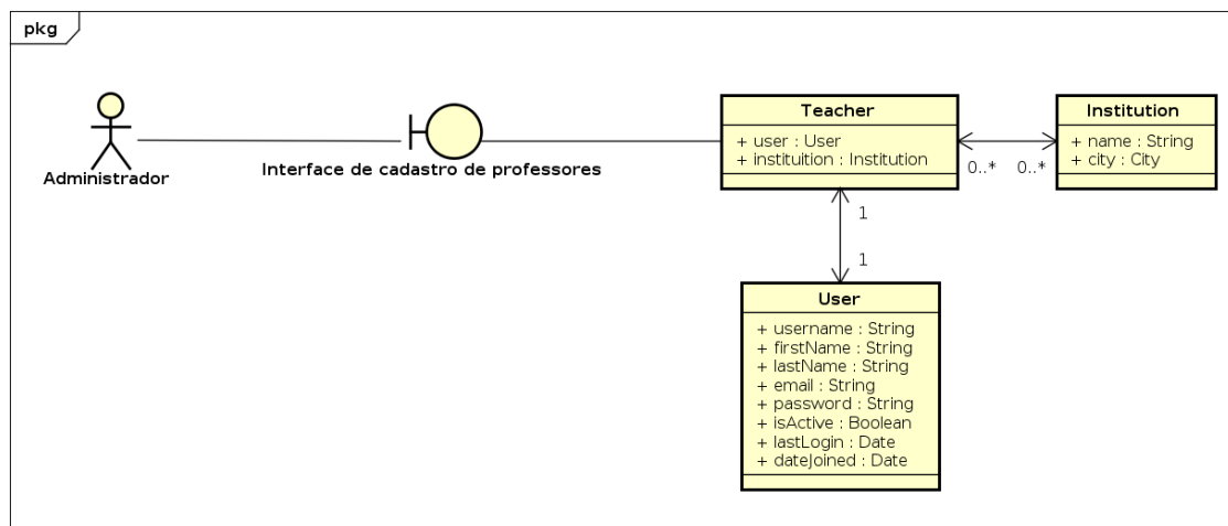
Figura 4.56: Diagrama de Robustez de Cadastro e Edição de Professores
