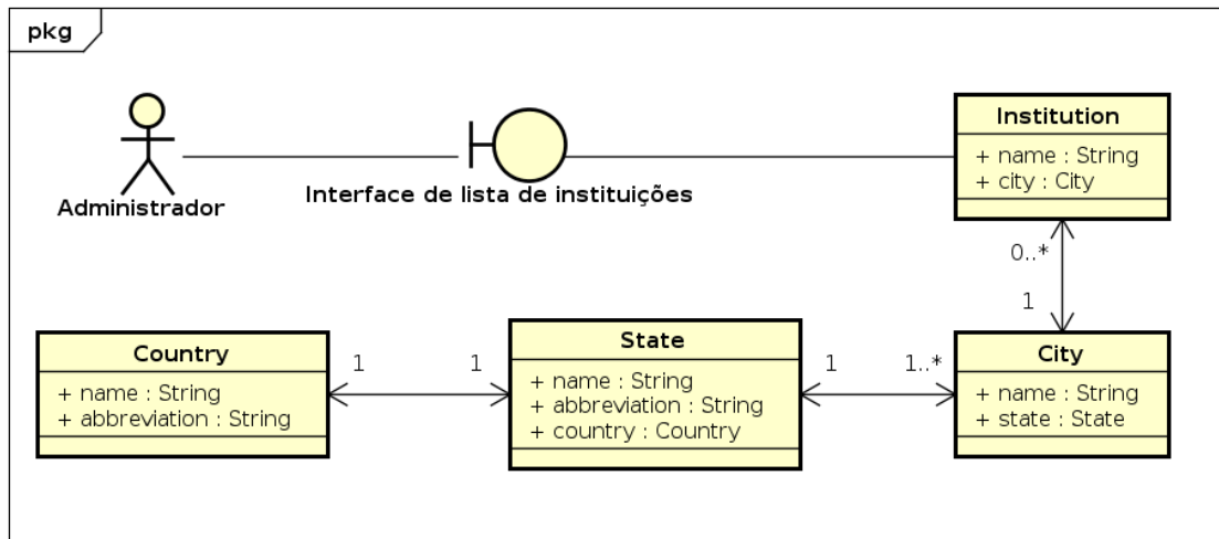
Figura 4.57: Diagrama de Robustez de Lista de Instituições
