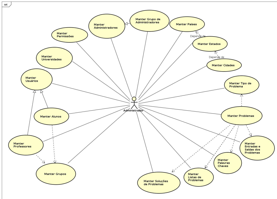
Figura 4.2: Casos de Uso que envolvem o ator Administrador
