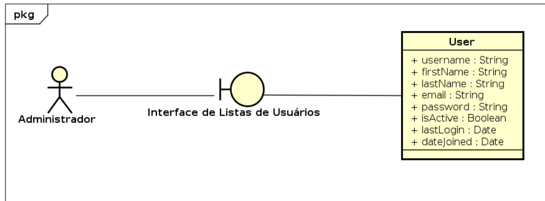
Figura 4.53: Diagrama de Robustez de Lista de Usuários
