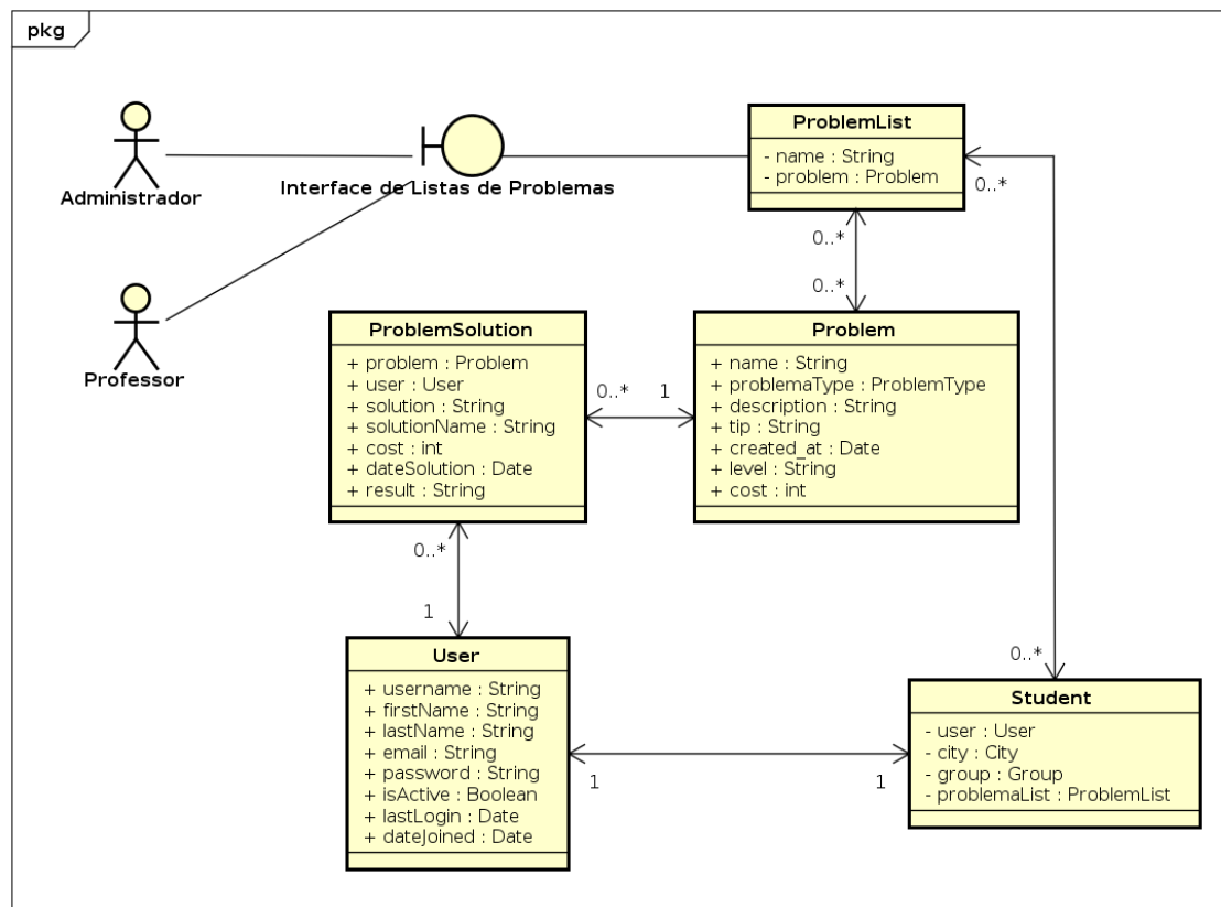
Figura 4.51: Diagrama de Robustez de Lista de Problemas
