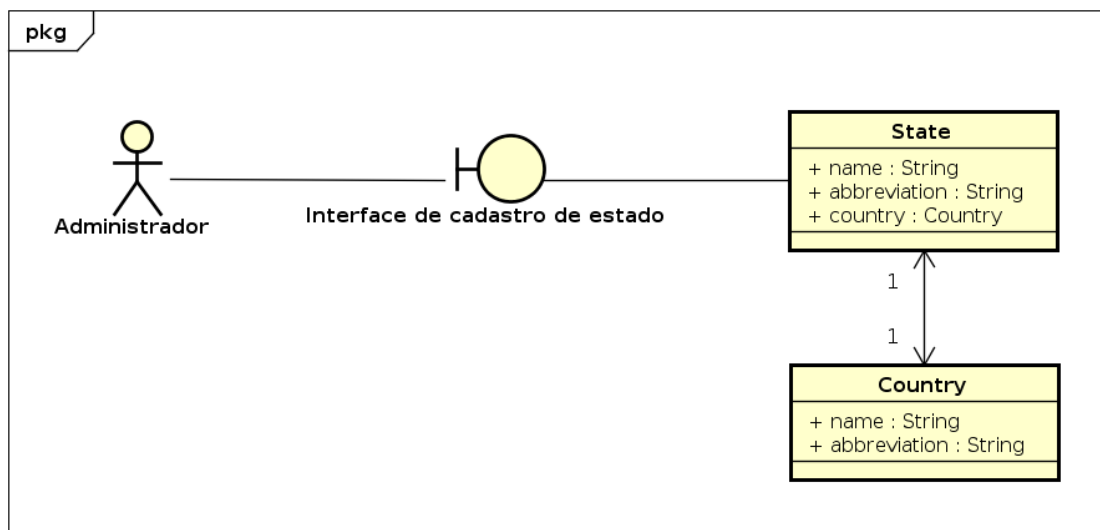
Figura 4.65: Diagrama de Robustez de Cadastro e Edição de Estado
