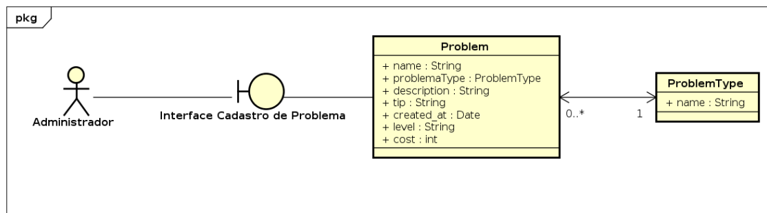
Figura 4.41: Diagrama de Robustez de Cadastro e Edição de Problema
