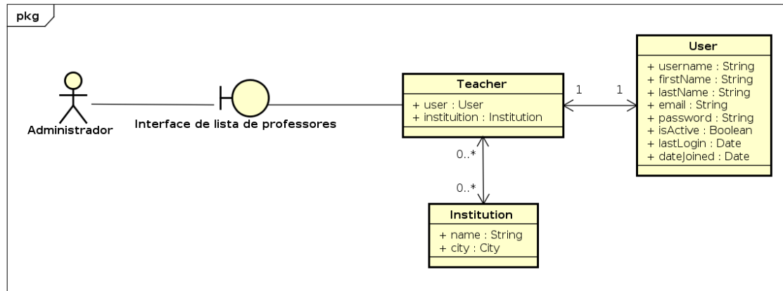
Figura 4.55: Diagrama de Robustez de Lista de Professores
