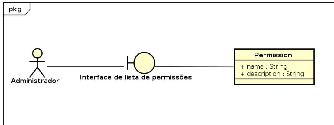
Figura 4.59: Diagrama de Robustez de Lista de Permissões
