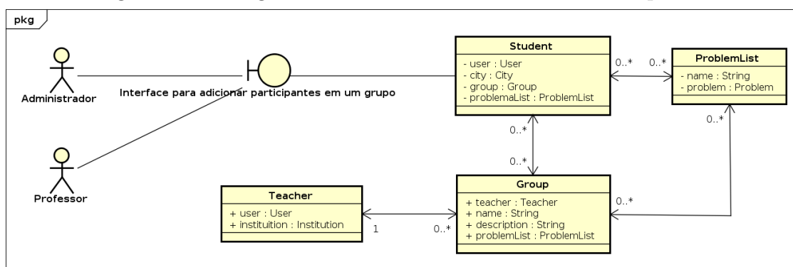
Figura 4.47: Diagrama de Robustez de Adicionar Participantes
