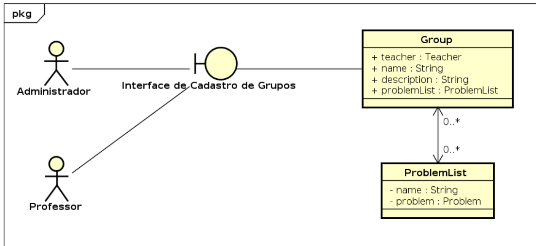
Figura 4.46: Diagrama de Robustez de Cadastro e Edição de Grupo
