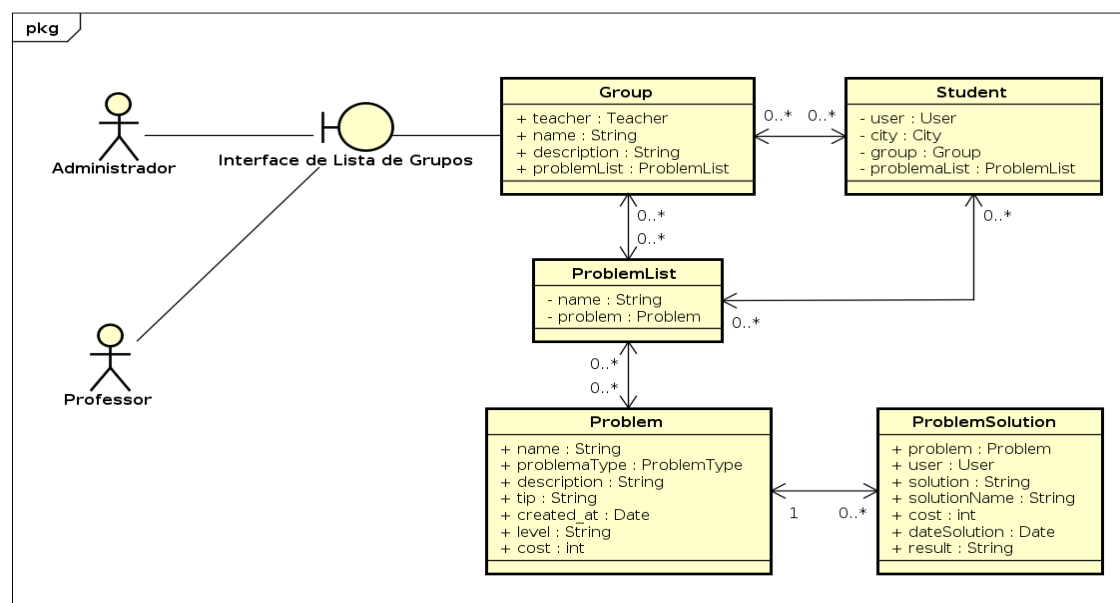
Figura 4.45: Diagrama de Robustez de Lista de Grupos
