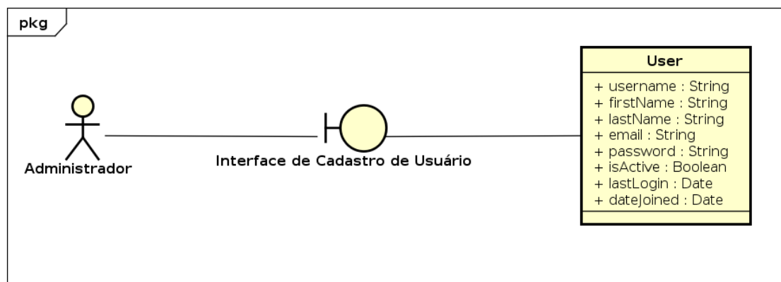
Figura 4.54: Diagrama de Robustez de Cadastro e Edição de Usuários
