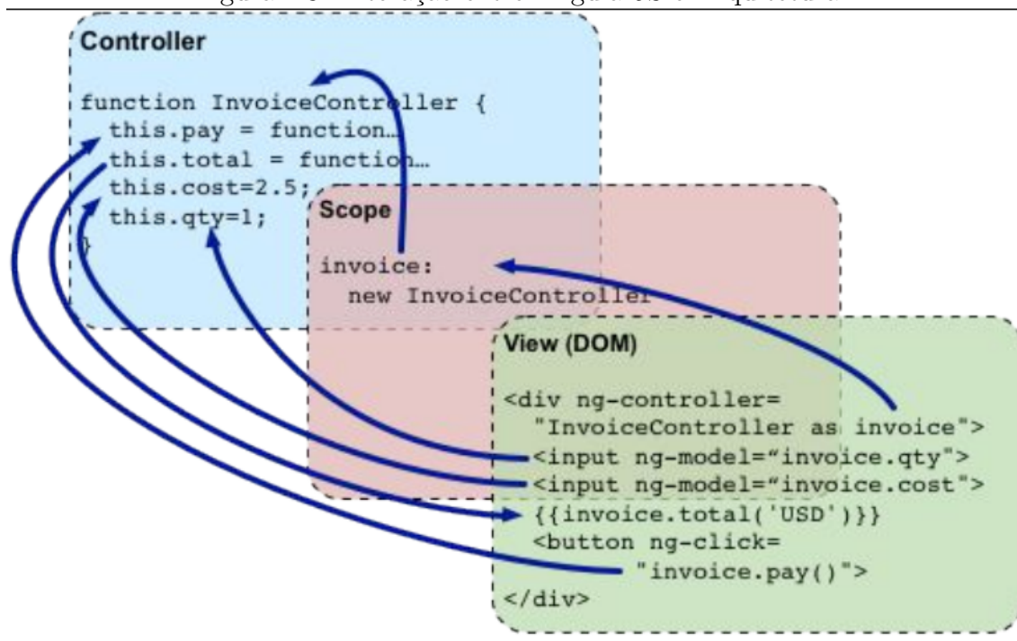
Figura 2.8: Interação entre AngularJS e Arquitetura
