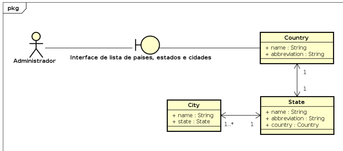
Figura 4.63: Diagrama de Robustez de Lista de Países, Estados e Cidades
