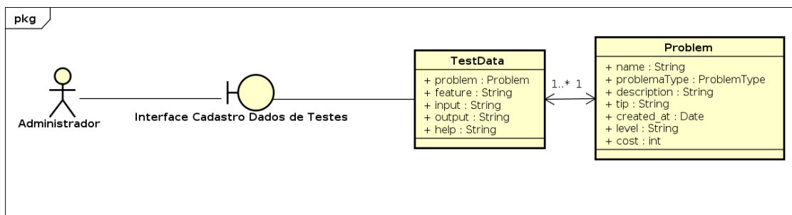
Figura 4.43: Diagrama de Robustez de Dados de Testes
