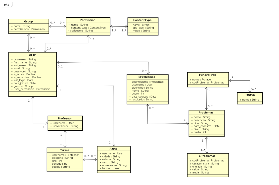
Figura 3.1: Diagrama de Domínio do Portal de Algoritmos Atual
