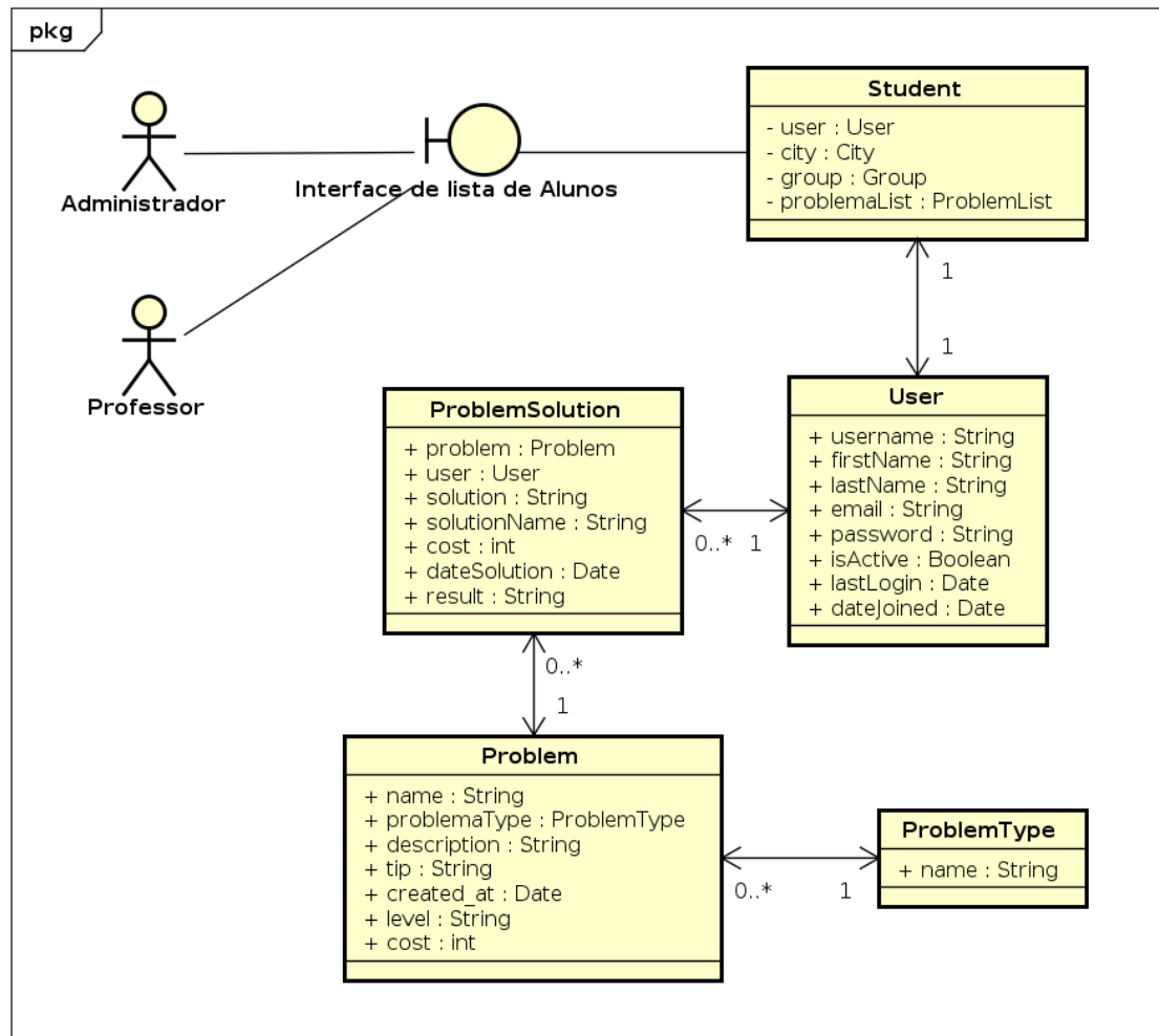
Figura 4.49: Diagrama de Robustez de Lista de Alunos
