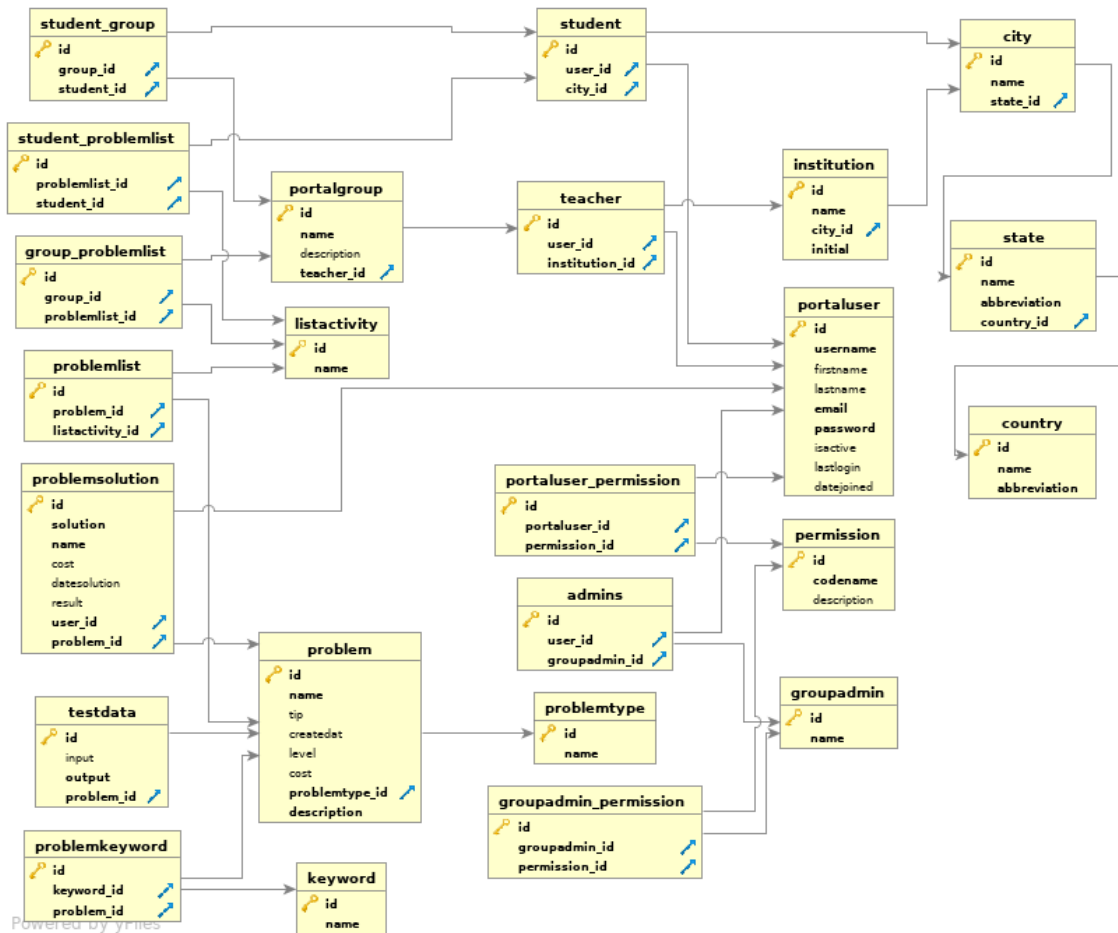
Figura 4.1: Diagrama de Domínio do Portal de Algoritmos Novo
