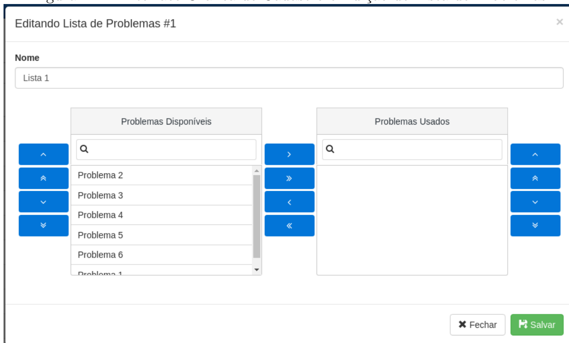
Figura 4.21: Interface Gráfica de Cadastro e Edição de Lista de Problemas
