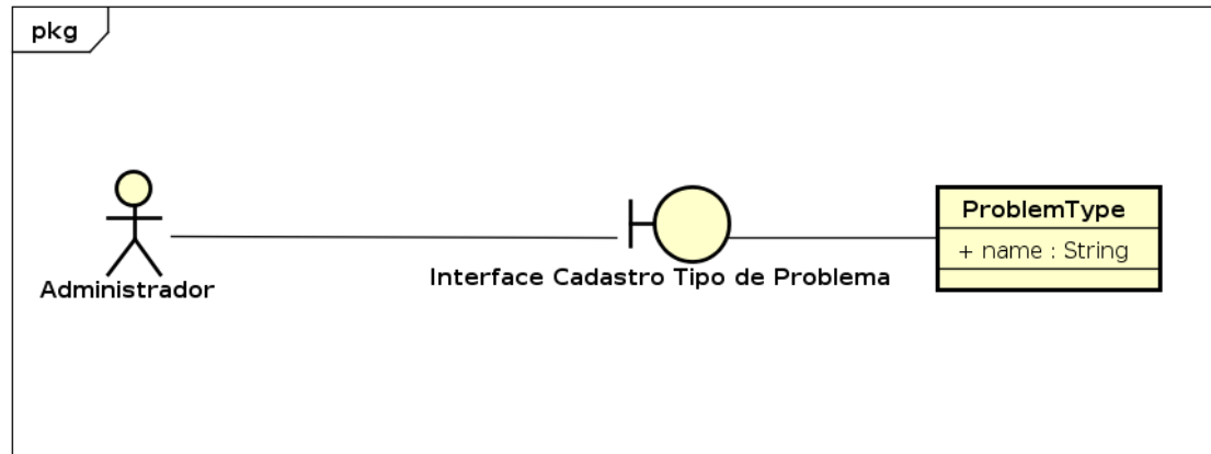
Figura 4.40: Diagrama de Robustez de Tipo de Problema
