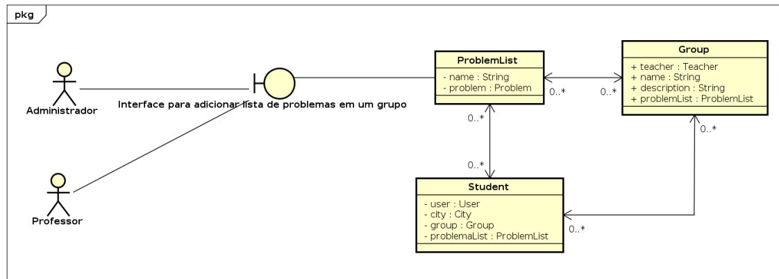
Figura 4.48: Diagrama de Robustez de Adicionar Lista de Problemas
