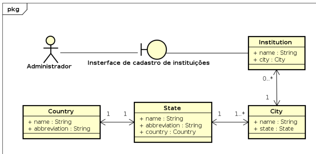
Figura 4.58: Diagrama de Robustez de Cadastro e Edição de Instituições
