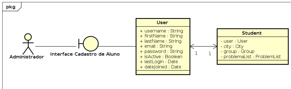
Figura 4.50: Diagrama de Robustez de Cadastro de Alunos pelo Administrador
