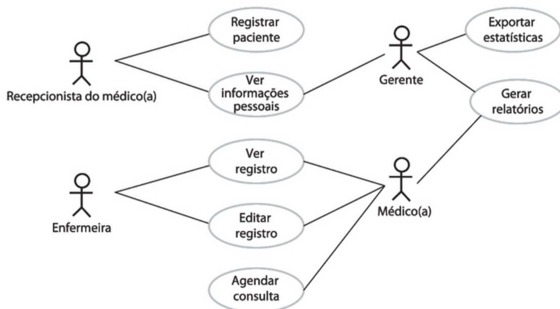
Figura 2.6: Casos de uso
