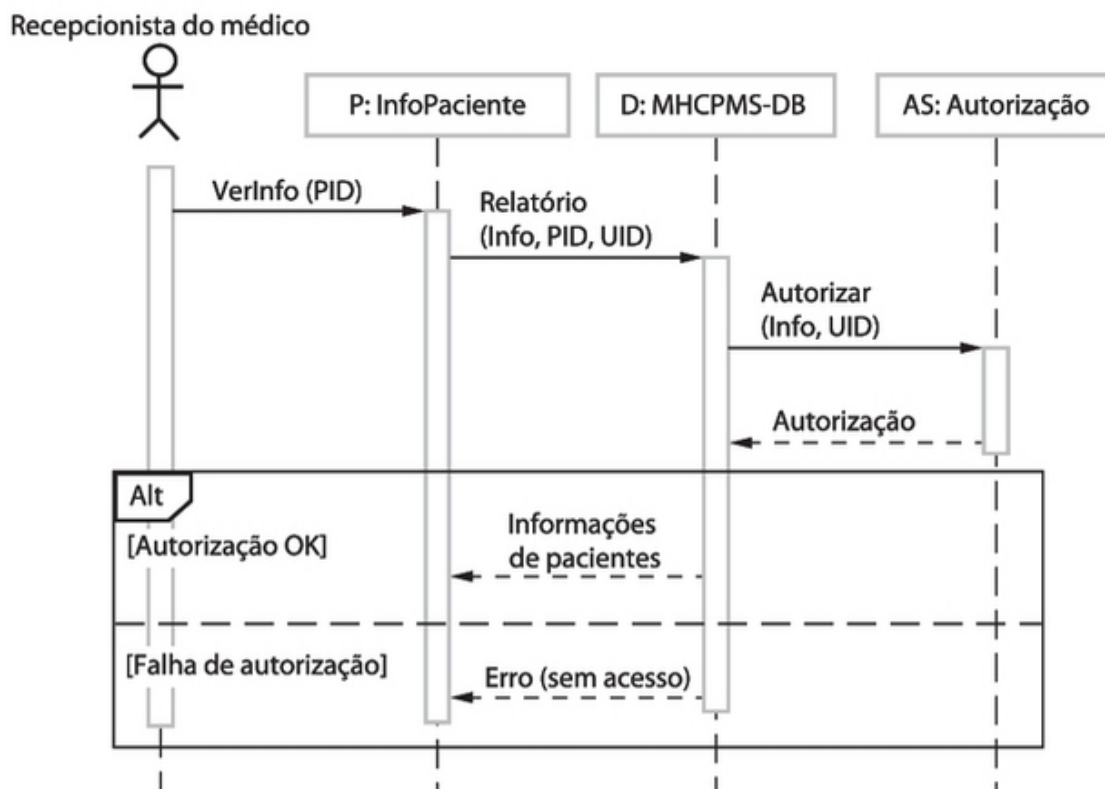
Figura 2.4: Diagrama de Sequência
