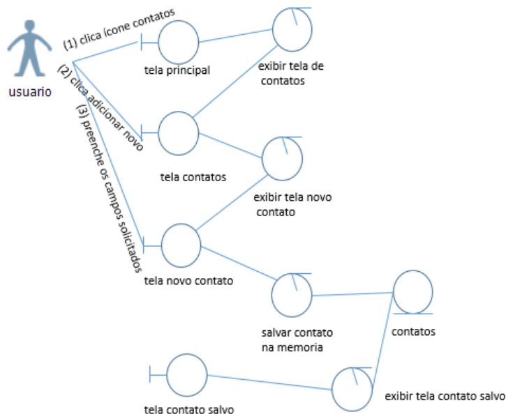
Figura 2.5: Diagrama e Robustez
