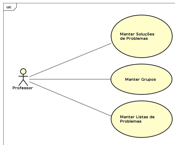
Figura 4.3: Casos de Uso que envolvem o ator Professor
