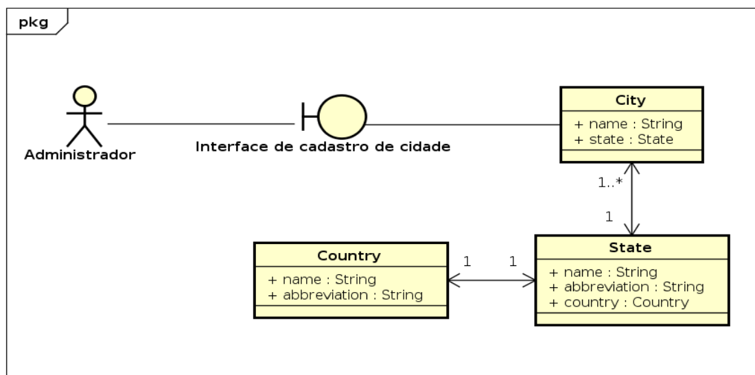
Figura 4.66: Diagrama de Robustez de Cadastro e Edição de Cidade
