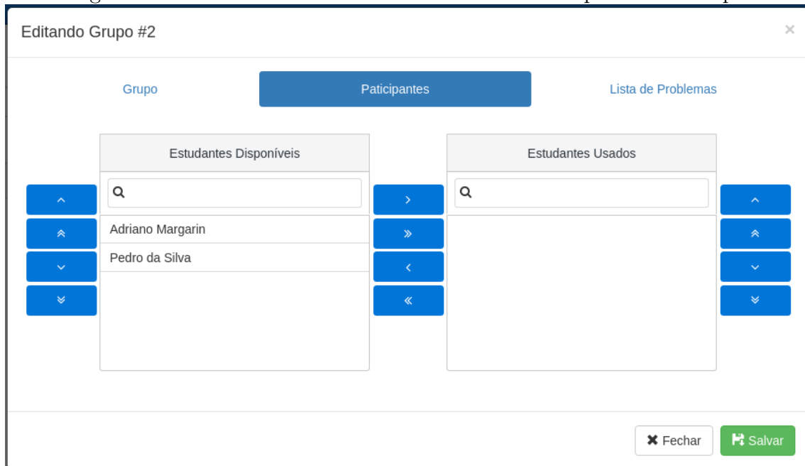
Figura 4.16: Interface Gráfica de Cadastro de Participantes no Grupo
