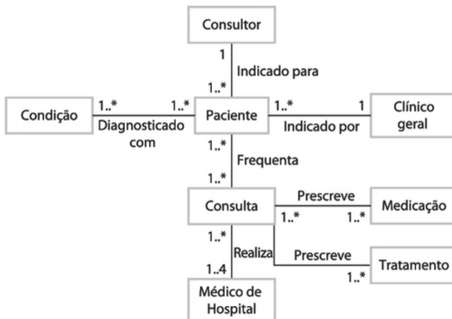
Figura 2.3: Diagramas de Classe
