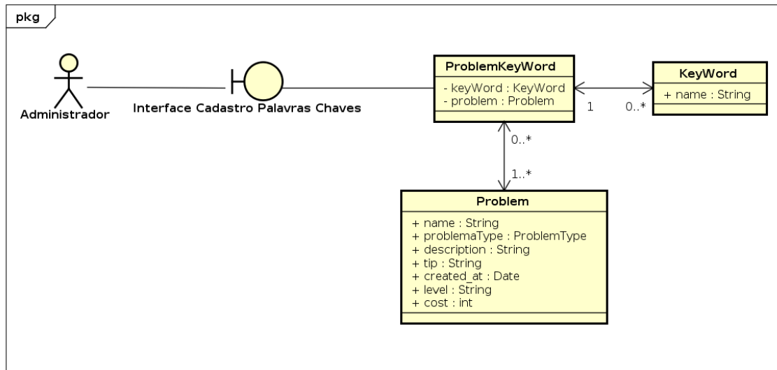
Figura 4.42: Diagrama de Robustez de Palavras-chave
