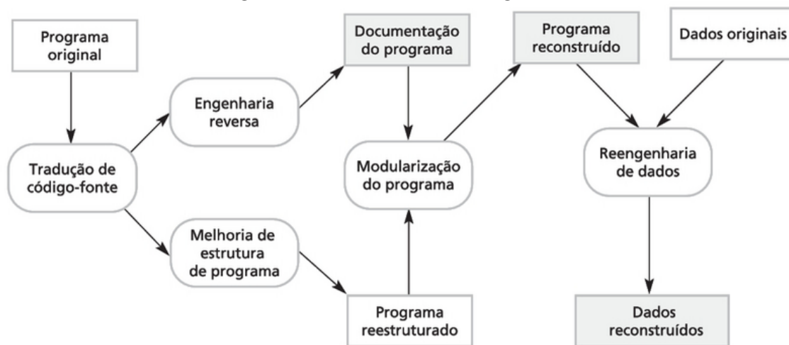
Figura 2.1: Processo de Reengenharia
