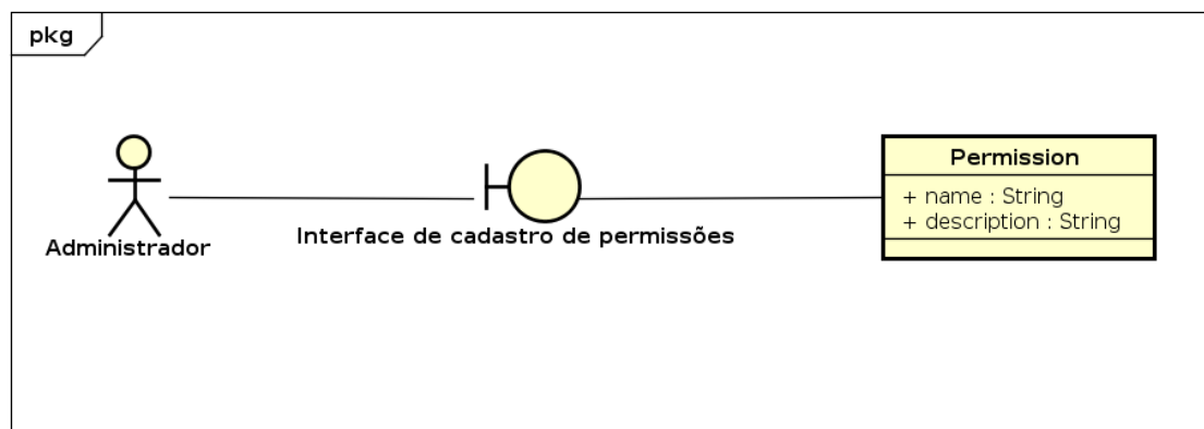
Figura 4.60: Diagrama de Robustez de Cadastro e Edição de Permissões
